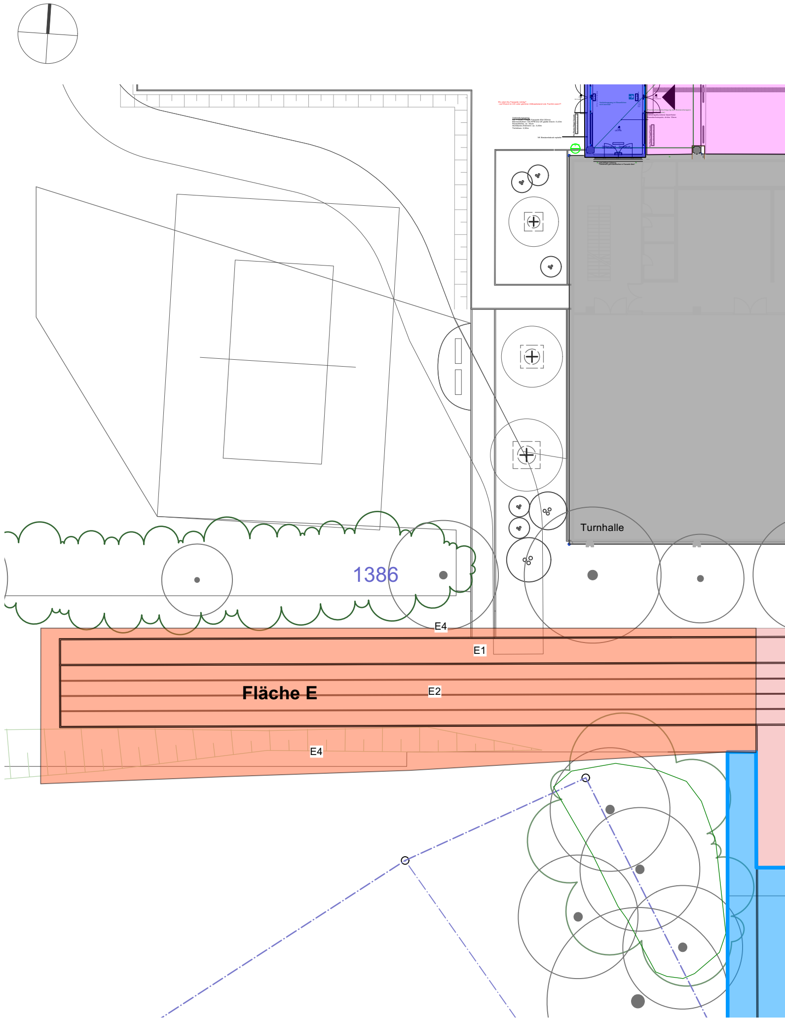
Abflusswirksame Flächen, Fläche E - Rigole 5
